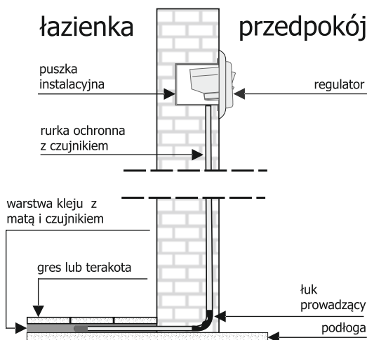
rys.11 rurka ochronna czujnika
