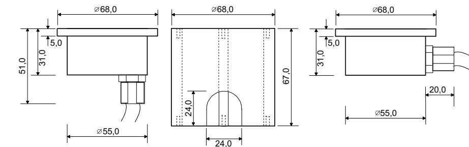
rzut boczny czujnika TC 3351 rzut boczny tulei do czujnika rzut boczny czujnika TC 3352
